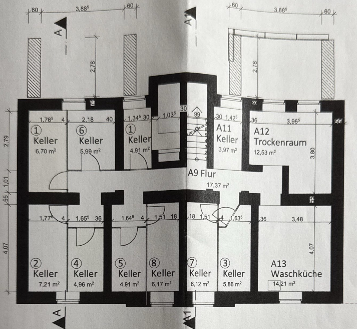
Grundriss Kellergeschoss, M.1:100
